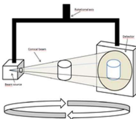
Slika 19. Prikaz načina rada CBCT uređaja.
